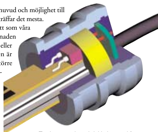
Trycktät givarhuvud, dubbel utsignal för redundans och mycket liten inbyggnadsmått – den ideala givaren för cylindrar.
